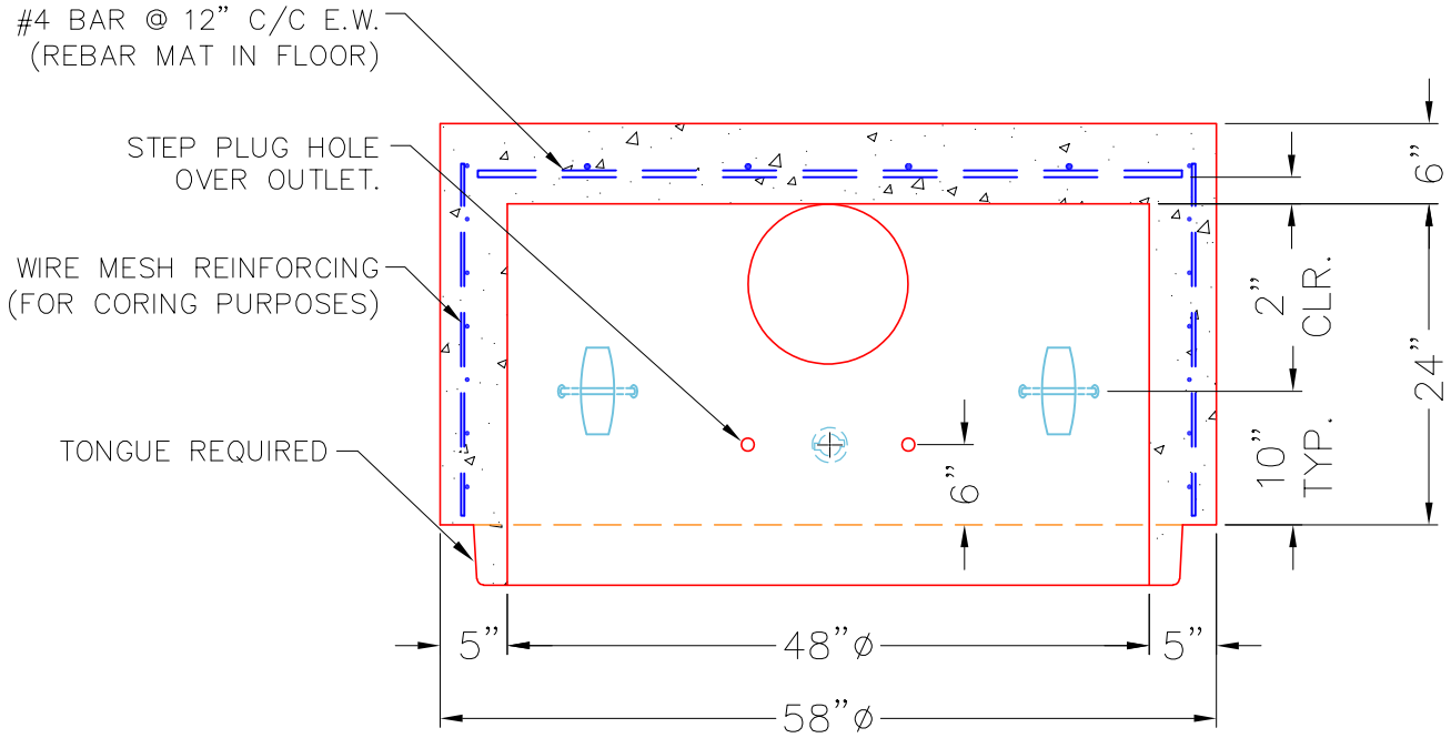
SECTION A-A
