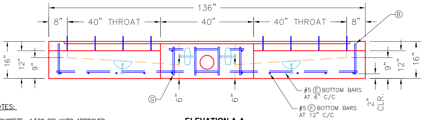
ELEVATION A-A
