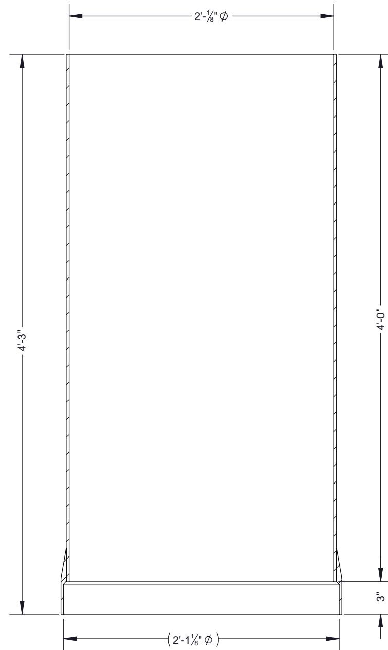
SECTION A-A
