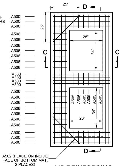
LID REINFORCING
