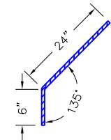
#5 (D) BENT BAR STUB
