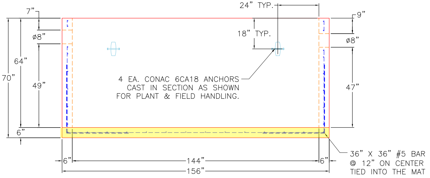
SECTION A-A
